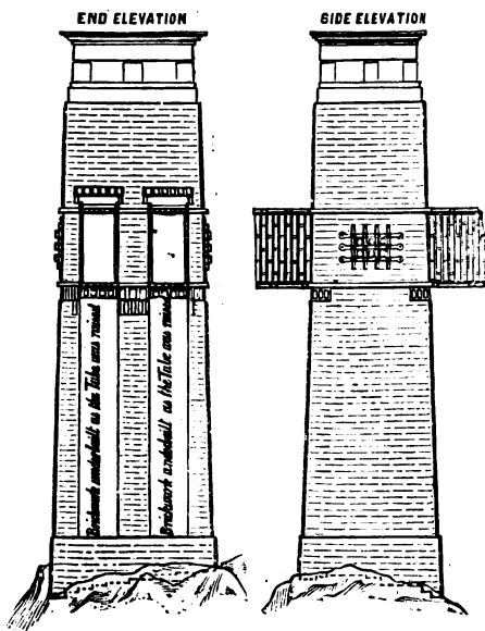
FIG. 98.—Britannia Tower.
