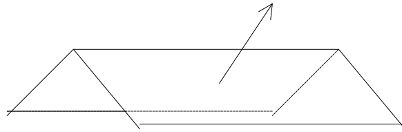
FIGURA 5: Vector ortogonal a una de las caras del diedro y con orientación hacia el exterior. Definimos el ángulo de un diedro como el ángulo de dos vectores asociados u ortogonales a cada uno de los planos del diedro y sentido u orientación a semiespacios (de los que divide el diedro al espacio) distintos.
