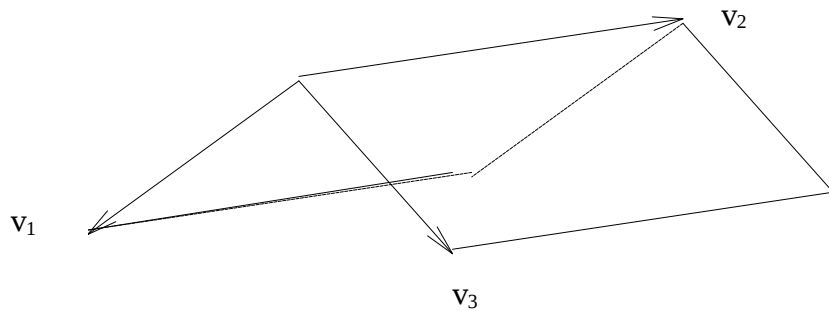
Figura 7: Diedro definido por tres vectores.
