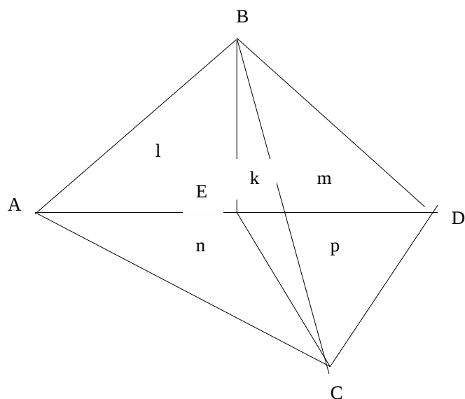
FIGURA 3: K^2 = PN - LM .
