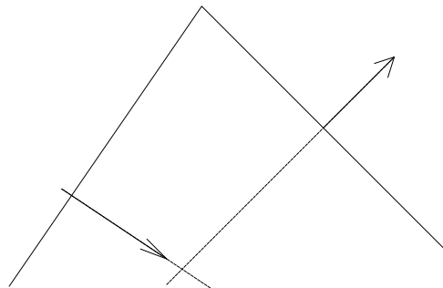
FIGURA 6: Sección normal del diedro, mostrando que el ángulo diedro es idéntico al que forman los vectores asociados a planos, uno interior y otro exterior al diedro.
